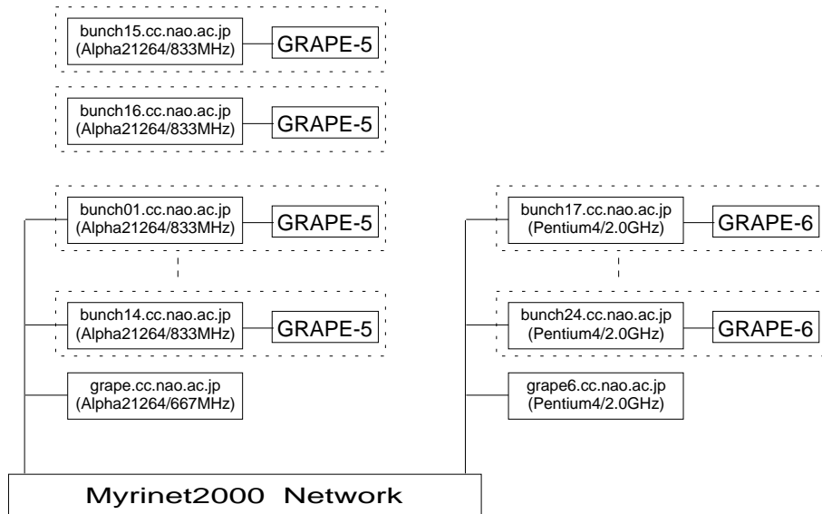
図 4.4: 国立天文台 GRAPE システム ネットワーク構成
